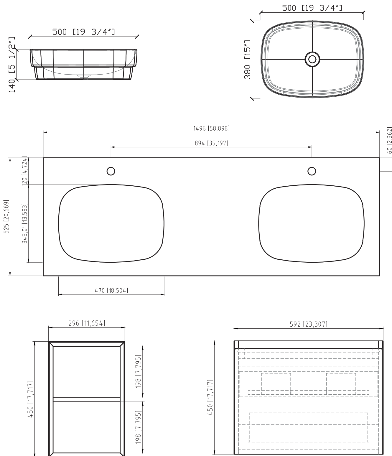
Vista Frontal de Modulo Central
