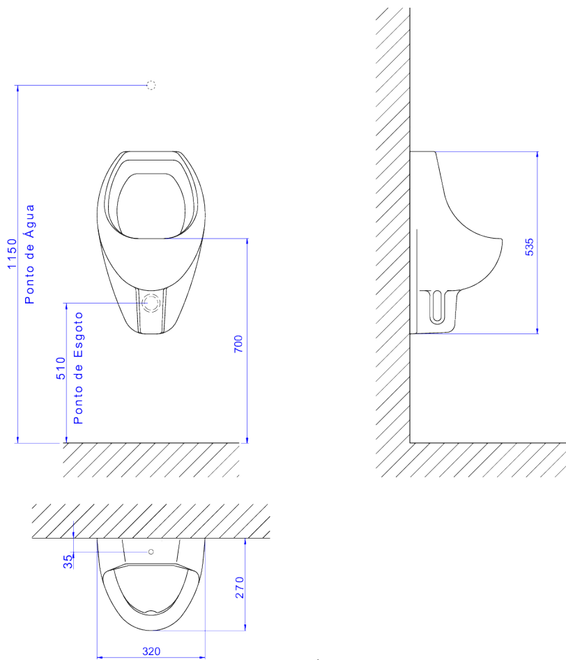
Desenho Técnico
