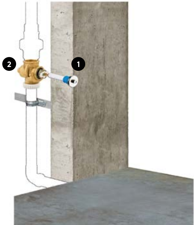
2 Válvula de descarga anti-vandálica leed. alta presión
