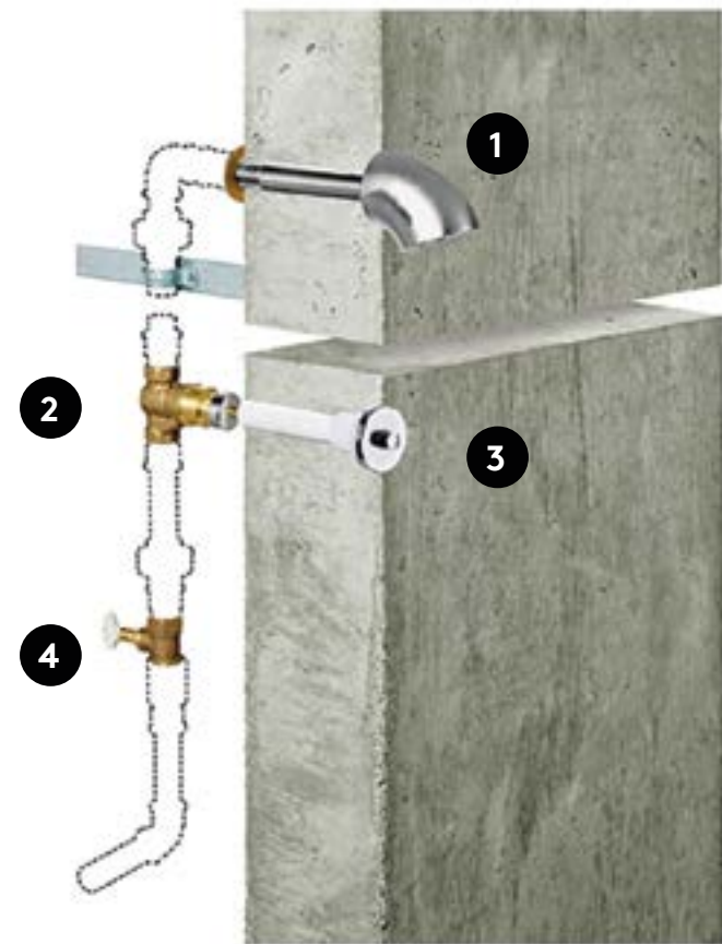
1 Ducha pasante de alta seguridad accionamiento hidro-mecánico
